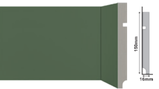
496 RP/Eucalipto Eucalyptus Cód. | Code - 29016
