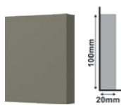
Sócalo 177 Cinza Titanium PLinth Block Titanium Gray Zócalin Gris Titanio
