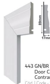
442 GN/BR Door Case White Contramarco Blanco Cód. | Code - 20006
