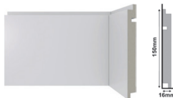
461 RP/BR Skirting Board White | Zócalo Blanco Cód. | Code - 20247
