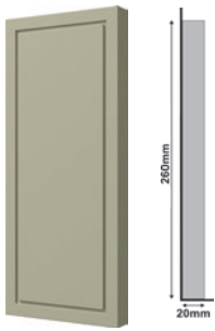
Sócalo 196 Cinza Glacial Plinth Block Glacial Gray Zócalin Gris Glacial 110 x 260 x 20mm Cód. | Code - 27536
