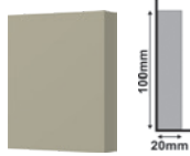
Sócalo 177 Cinza Glacial PLinth Block Glacial Gray Zócalin Gris Glacial
