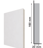
Sócalo 187 Plinth Block | Zócalin 110 x 160 x 20mm Cód. | Code - 27377
