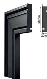
3444 GN/Black Door Case Black Contramarco Negro Cód. | Code - 26447
