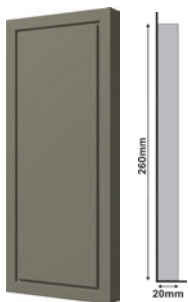
Sócalo 196 Cinza Titanium Plinth Block Titanium Gray Zócalin Gris Titano 110 x 260 x 20mm Cód. | Code - 27528
