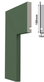
547 GN/Eucalipto Eucalyptus Eucalipto Cód. | Code - 29022
