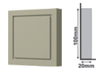
Roseta 193 Cinza Glacial Rosette Glacial Gray Roseta Gris Glacial 100 x 100 x 20mm Cód. | Code - 27533
