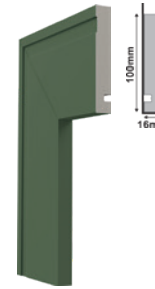
457 GN/Eucalipto Eucalyptus Eucalipto Cód. | Code - 28910
