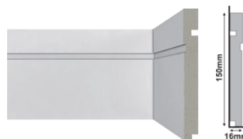
503 RP/BR Skirting Board White | Zócalo Blanco Cód. | Code - 25427
